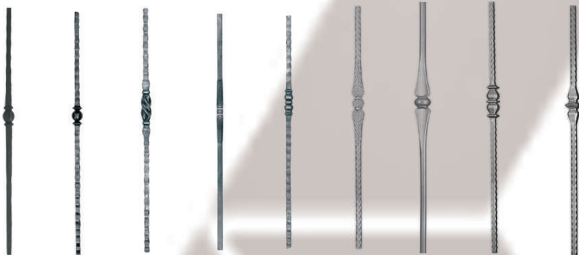
03-024 03-030 03-031 03-032 03-033 03-045 03-046 03-047 03-048 20 мм 25 мм 25 мм 25 мм 25 мм 24 мм 26 мм 24 мм 24 мм 1200 мм 1200 мм 1200 мм 1200 мм 1200 мм 1000 мм 1000 мм 1000 мм 1000 мм кована кована кована гладко кована кована усукан кована кована
