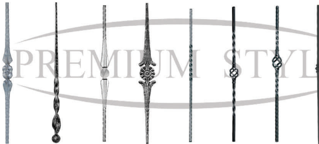
03-015 03-016 03-017 03-018 03-020 03-021 03-022 03-023 16 мм 16 мм 16 мм 14 мм 20 мм 20 мм 20 мм 20 мм 900 мм 900 мм 900 мм 900 мм 1100 мм 1200 мм 1200 мм 1200 мм кована кована кована кована кована torsiune кована кована
